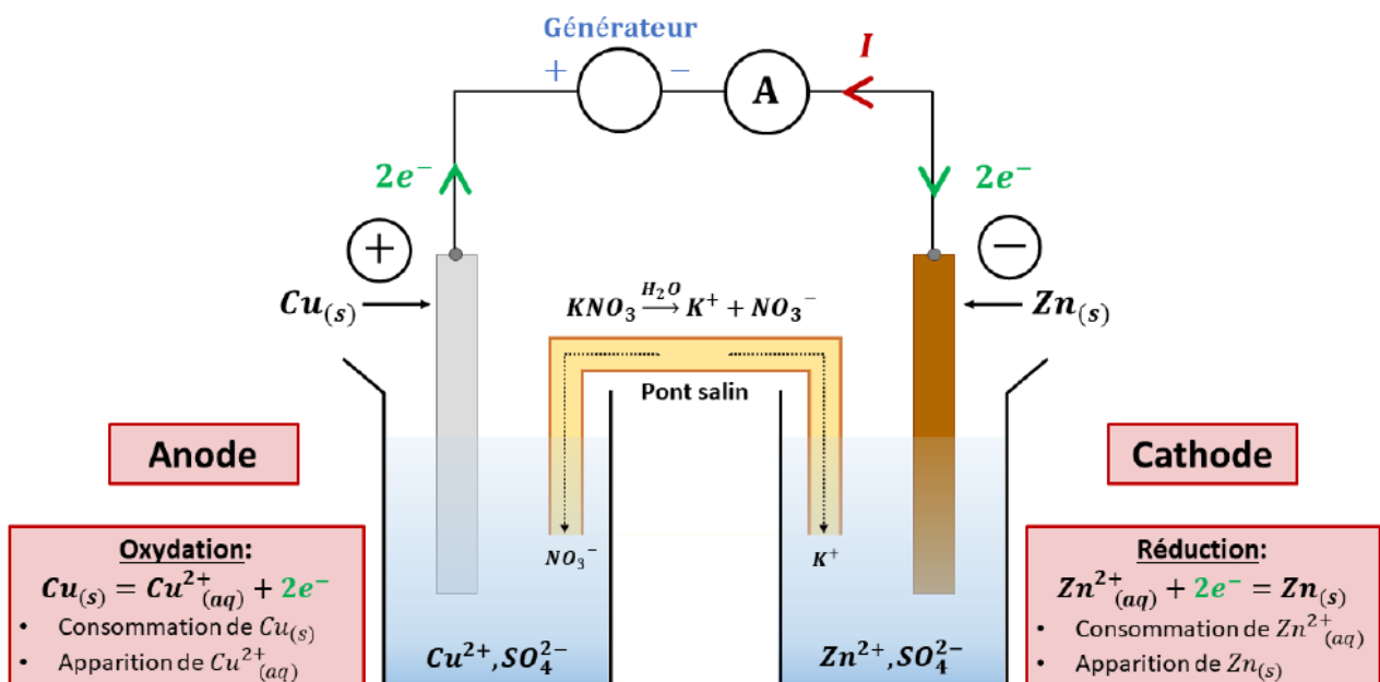
Figure 18.1 – Schéma de l'électrolyse associée à la pile Daniell vue au chapitre 4
